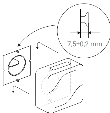
Рисунок 6.8. Навешивание устройства
