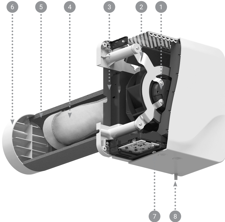
Рисунок 5.1. Состав системы:
