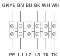
Схема 5 (400 В, 3 ф, 50 Гц.)
