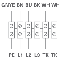
Схема 5 (400 В, 3 ф, 50 Гц.)
