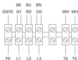
Схема 5 (400 В, 3 ф, 50 Гц.)
