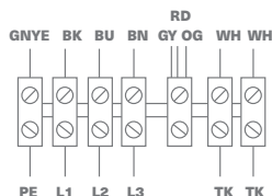
Схема 4 (400 В, 3 ф, 50 Гц.)
